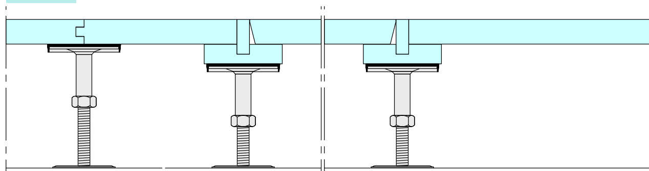
F181-V12 Revizioni otvor, otpornost na požar F30 / F60
