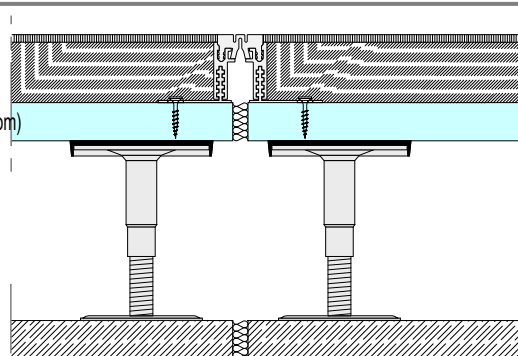
F181-V10 Primer: Montiranje pokretnog dilatacionog profila
