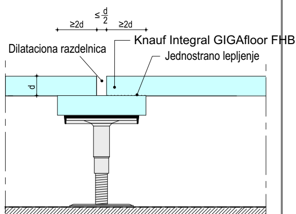
F181-V11 Dilataciona razdelnica sa podmetnutim slojem za zaštitu od požara
