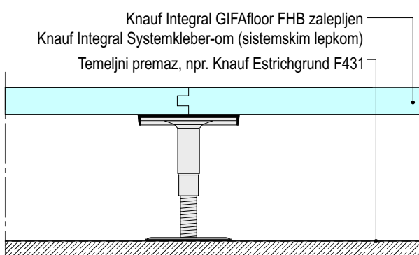
F181-V5 Pozicioniranje nožica ispod spoja elemenata
