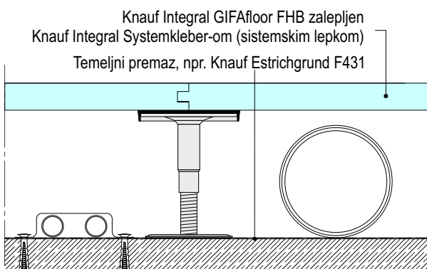
F181-V4 Korišćenje prostora podignutog poda za instalaciju
