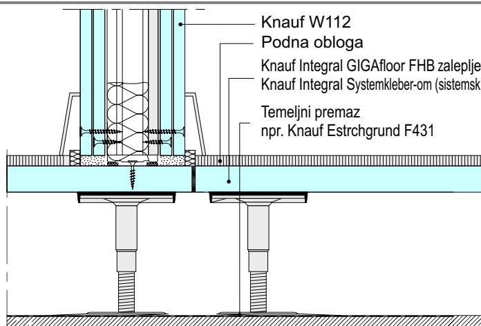
F181-V7 Laki pregradni zid na GIFAfloor FHB
